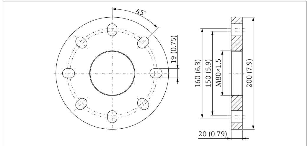
49 UNI 3"/DN80/80A 法兰，适用带空气吹扫接口的 PTFE 水滴型天线 (50 mm (2 in)口径)。测量单位 mm (in)
