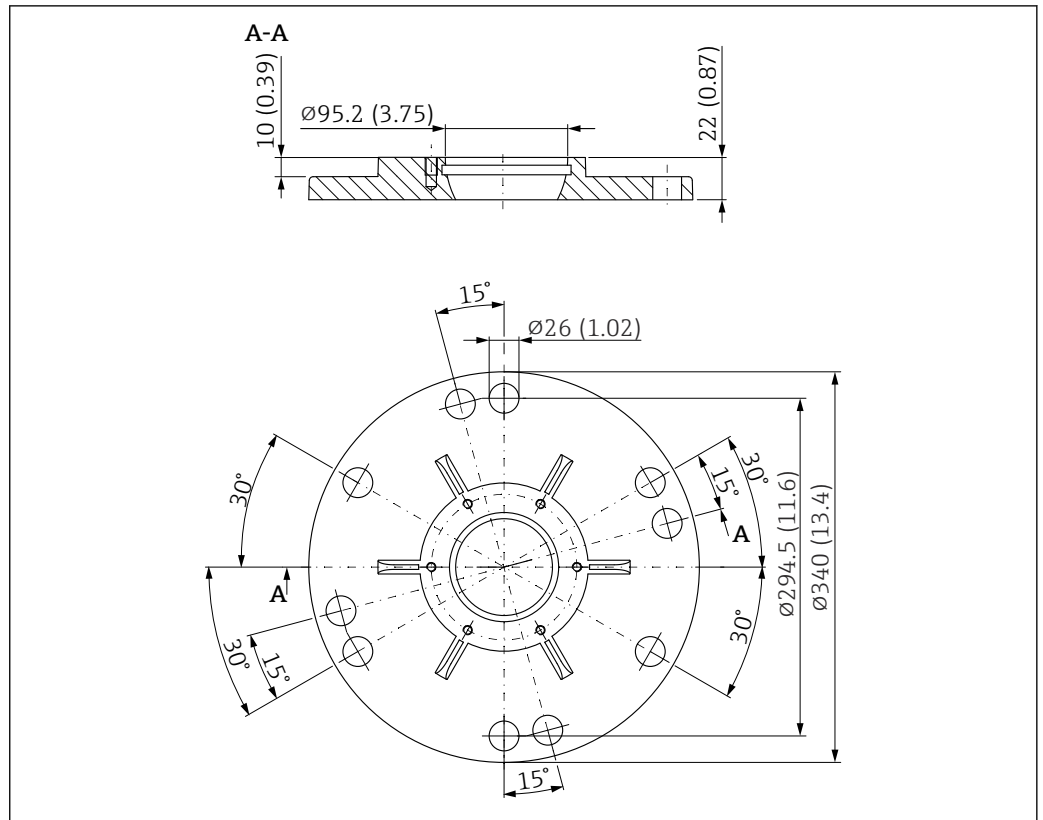
图 46 UNI 8"/DN200/200A 法兰的外形尺寸示意图; 适用带天线角度调节装置的天线。测量单位 mm (in)
