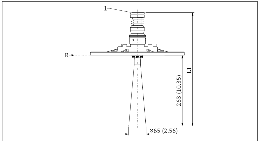
43 DN65 喇叭天线的外形尺寸示意图；带 UNI 法兰和天线角度调节装置。测量单位 mm (in)
