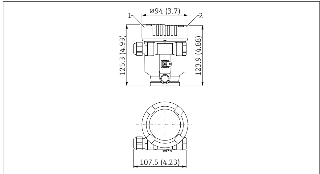
图 37 单腔室塑料 (PBT) 外壳的外形尺寸示意图。测量单位 mm (in)
