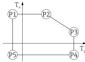
35 316L 外壳, 卫生型; 过程温度: -40 ... +280 °C (-40 ... +536 °F)
