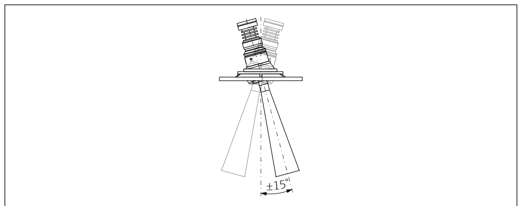
8 喇叭天线，带天线角度调节装置
