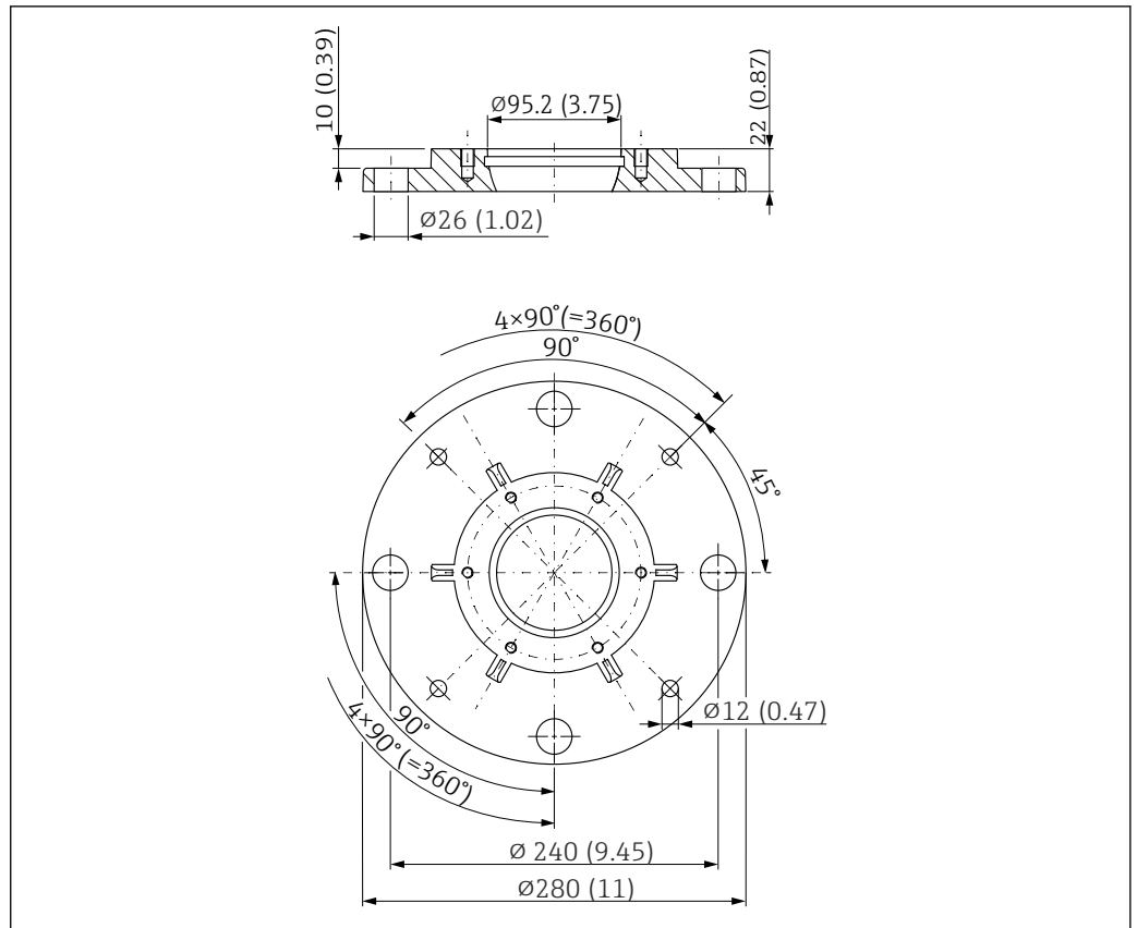
图 58 UNI 6"/DN150/150A 法兰的外形尺寸示意图; 适用带角度调节装置的天线。测量单位 mm (in)
