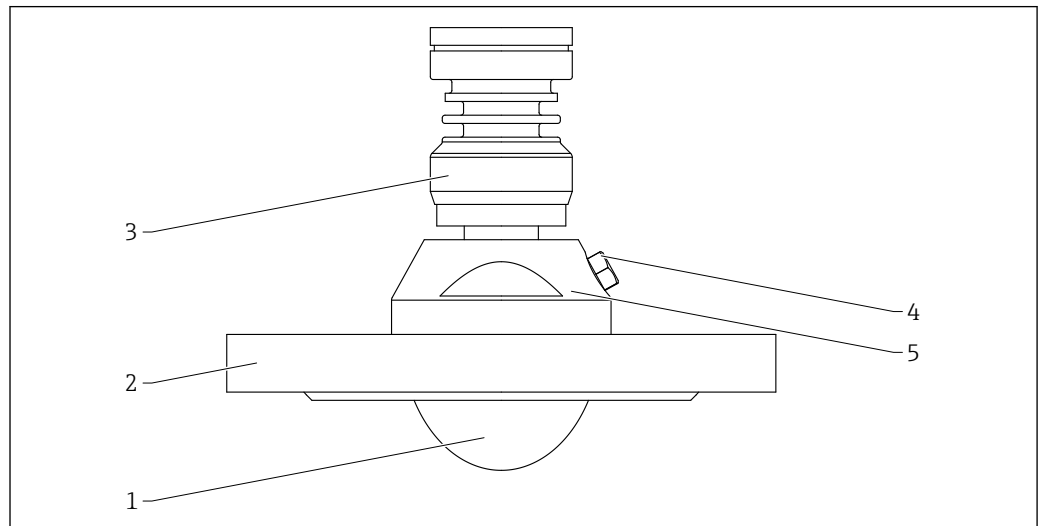
图 64 齐平安装天线（80 mm (3 in) 口径）的材质；带法兰和空气吹扫接口。测量单位 mm (in)
