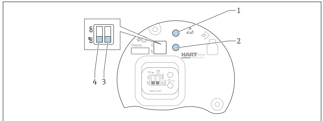
图 67 HART 电子插件上的操作按键和 DIP 开关
