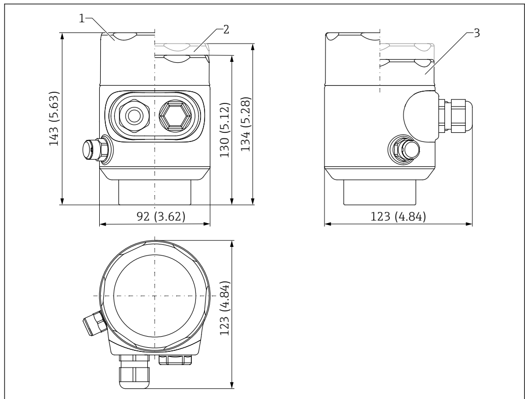
图 39 316L 单腔室外壳 (卫生型) 的外形尺寸示意图。测量单位 mm (in)
