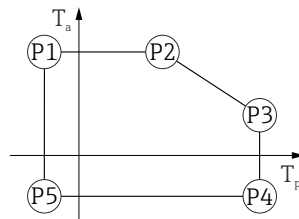
36 316L 外壳, 卫生型; 过程温度: -40 ... +450 °C (-40 ... +842 °F)
