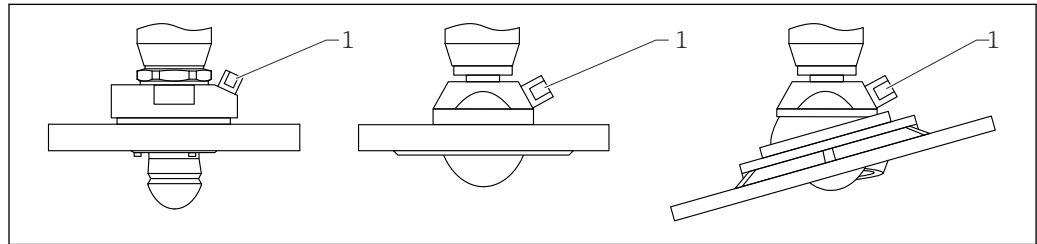
图 10 天线，带空气吹扫接口
