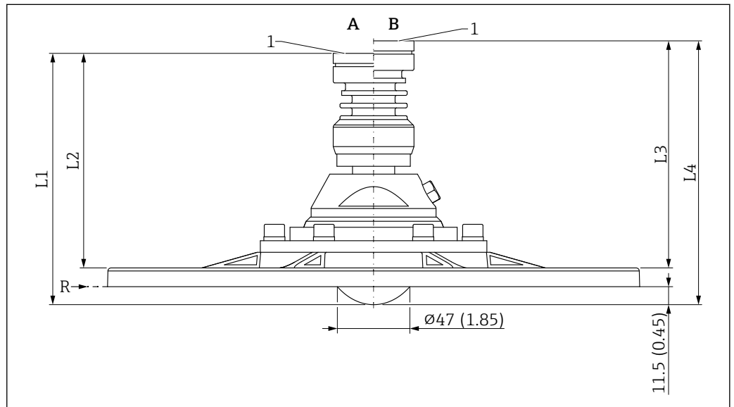
56 齐平安装天线 (80 mm (3 in)口径) 的外形尺寸示意图; 带 UNI 法兰、天线角度调节装置和空气吹扫接口。测量单位 mm (in)
