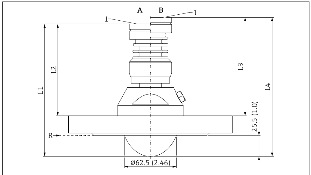
图 52 PTFE 齐平安装天线 (80 mm (3 in)口径) 的外形尺寸示意图; 带标准法兰和空气吹扫接口。测量单位 mm (in)
