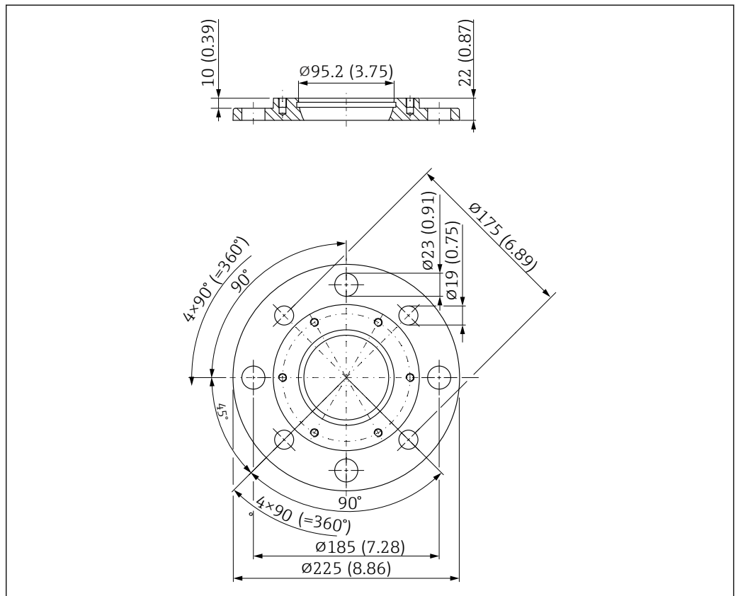
44 UNI 4"/DN100/100A 法兰的外形尺寸示意图；适用带天线角度调节装置的天线。测量单位 mm (in)
