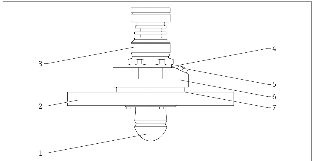
图 63 水滴型天线的材质；带空气吹扫接口。测量单位 mm (in)
