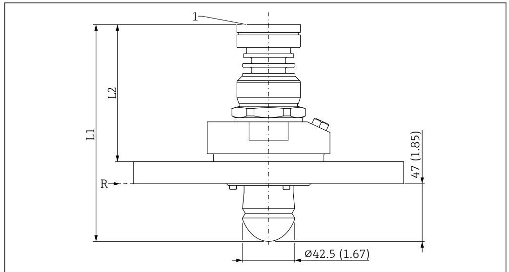
48 PTFE 水滴型天线 (50 mm (2 in)口径) 的外形尺寸示意图; 带 UNI 法兰和空气吹扫接口。测量单位 mm (in)
