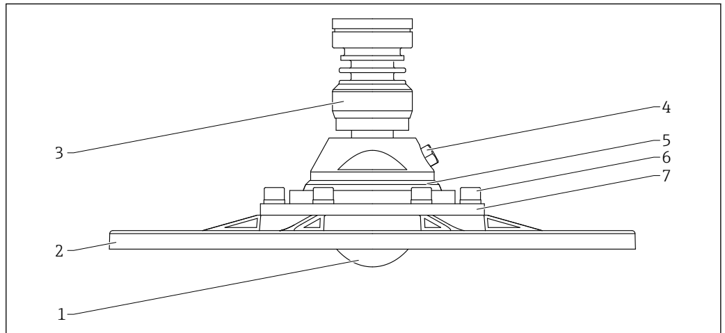
图 66 齐平安装天线 (80 mm (3 in)口径) 的材质; 带 UNI 法兰、天线角度调节装置和空气吹扫接口
