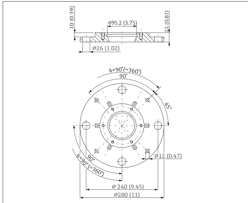
图 45 UNI 6"/DN150/150A 法兰的外形尺寸示意图；适用带角度调节装置的天线。测量单位 mm (in)
