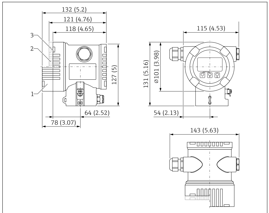
图 40 双腔室外壳的外形尺寸示意图。测量单位 mm (in)
