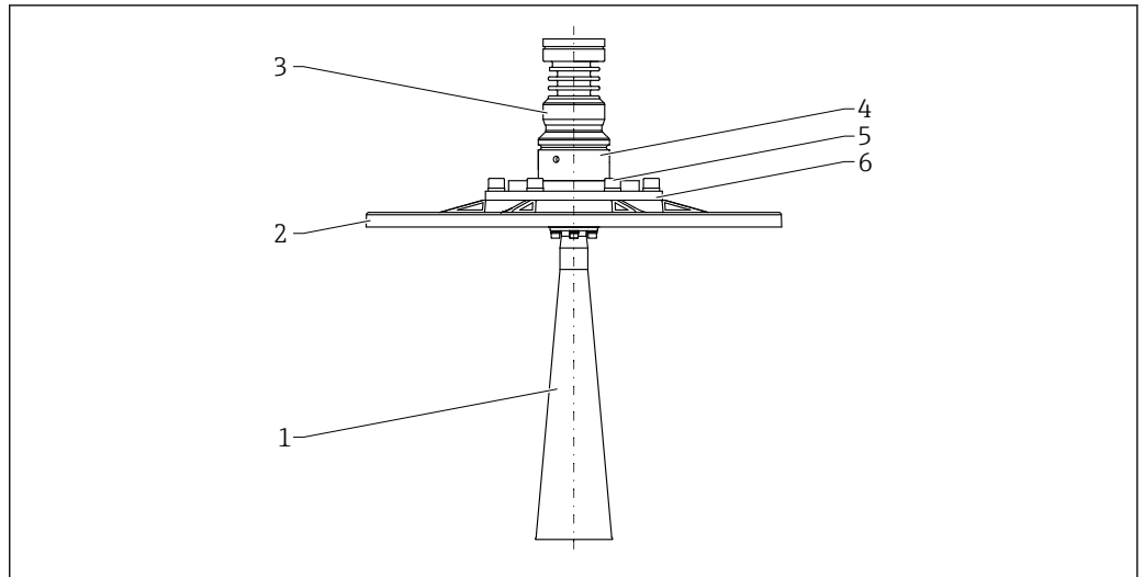
☐ 62 DN65 喇叭天线的材质; 带 UNI 法兰和天线角度调节装置。测量单位 mm (in)
