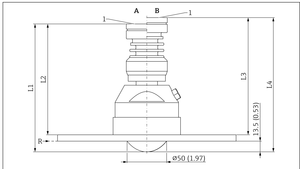
图 53 PTFE 齐平安装天线 (80 mm (3 in) 口径) 的外形尺寸示意图; 带 UNI 法兰和空气吹扫接口。测量单位 mm (in)
