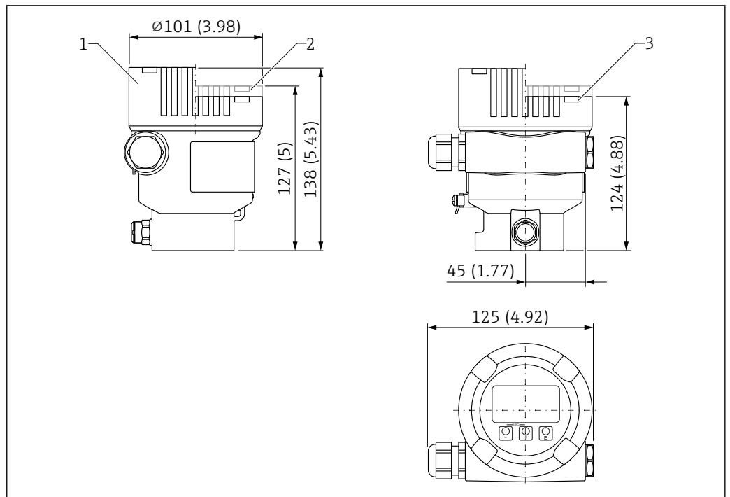
图 38 单腔室铝外壳的外形尺寸示意图。测量单位 mm (in)
