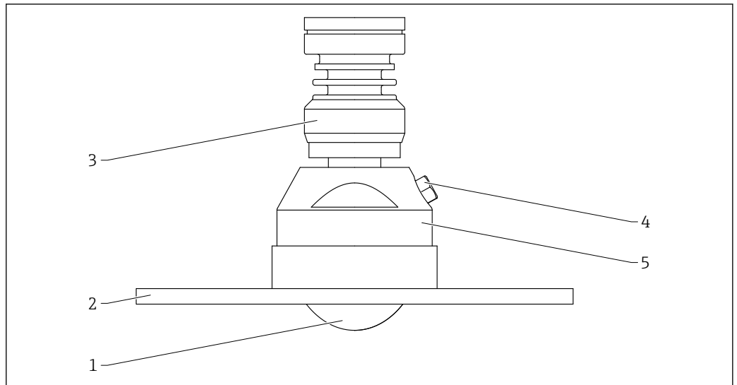
图 65 齐平安装天线 (80 mm (3 in)口径) 的材质，带 UNI 法兰和空气吹扫接口。测量单位 mm (in)
