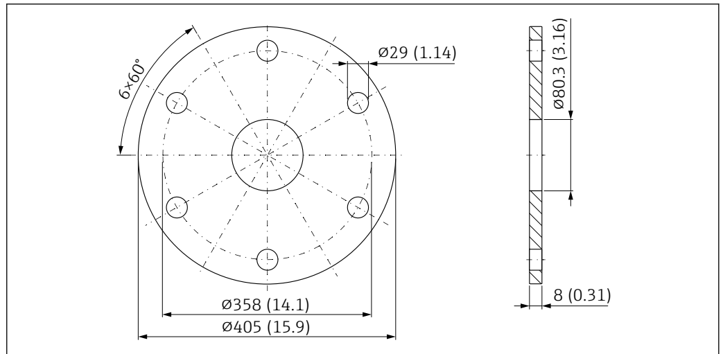
55 UNI 10"/DN250/250A 法兰的外形尺寸示意图; 适用带空气吹扫接口的 DN80 天线。测量单位 mm (in)
