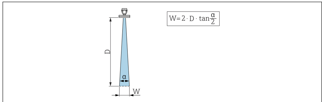
图 11 波束角 \alpha 、距离 D 和波束宽度 W 的相互关系
