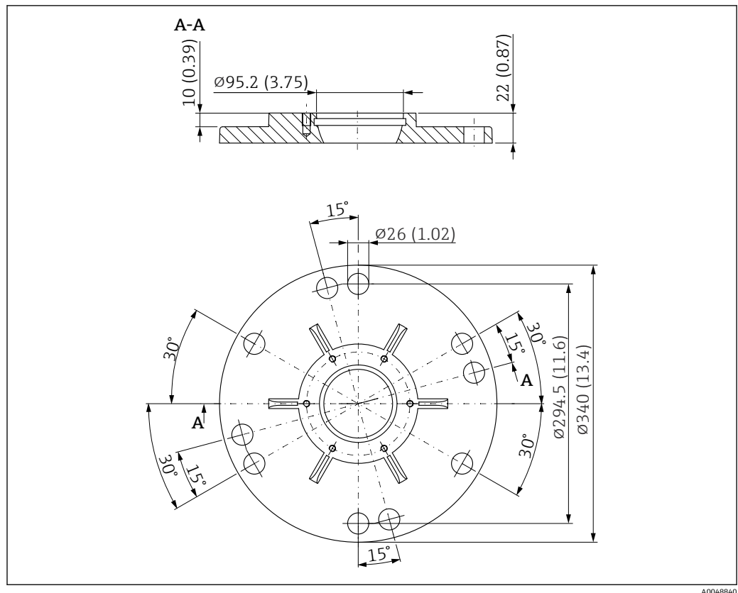
图 59 UNI 8"/DN200/200A 法兰的外形尺寸示意图；适用带天线角度调节装置的天线。测量单位 mm (in)
