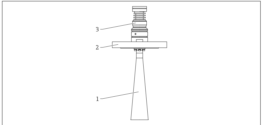
☐ 61 DN65 喇叭天线的材质。测量单位 mm (in)
