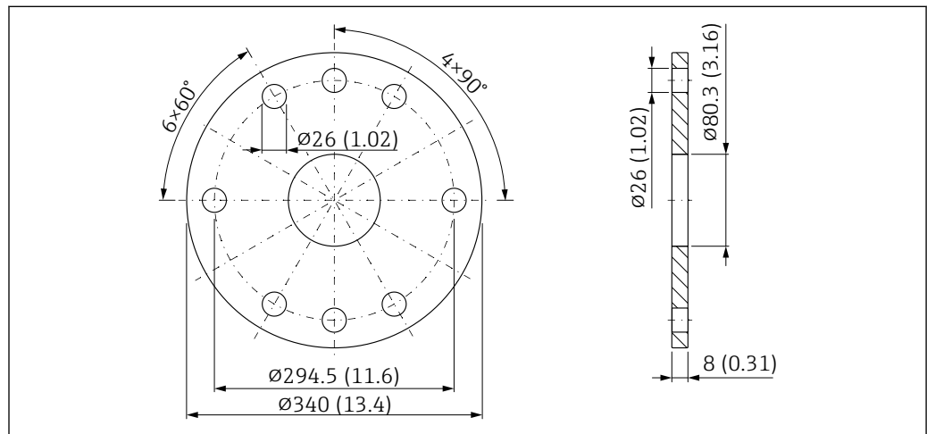
图 54 UNI 8"/DN200/200A 法兰的外形尺寸示意图; 适用带空气吹扫接口的 DN80 天线。测量单位 mm (in)
